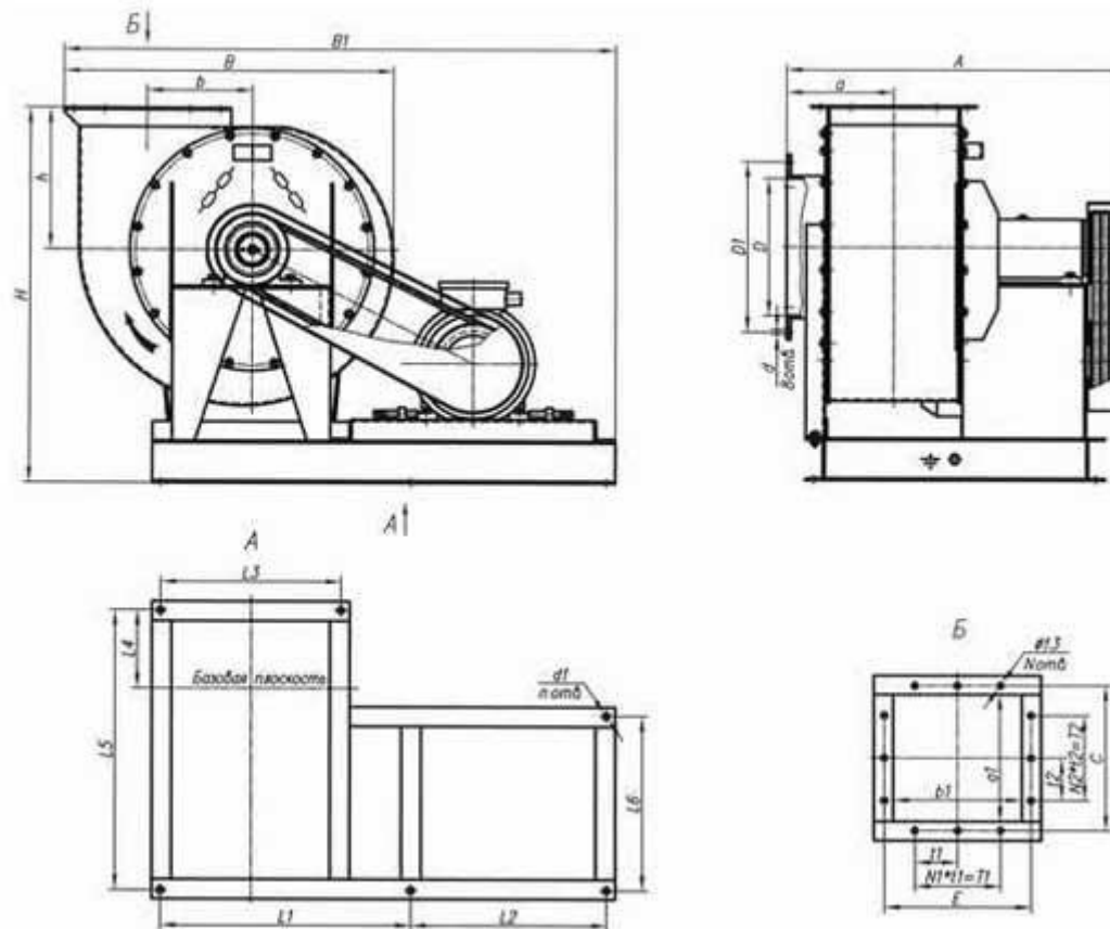
Рис.1. Габаритные размеры вентиляторов ЦП7-40
